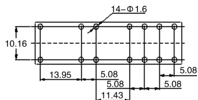
安装尺寸图 (底视图)
