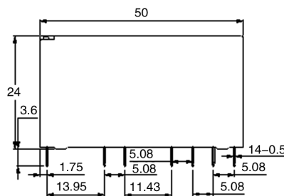
外形尺寸图
