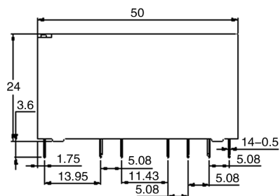
外形尺寸图
